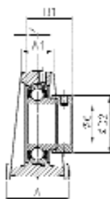
ESPAE200
