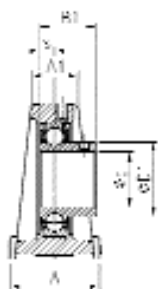
USPAE200
