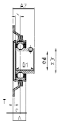
USPFE200
