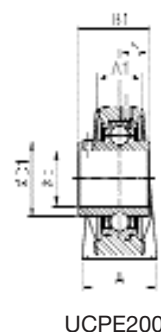
UCPE200
