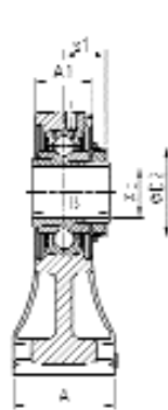
UKPH200H
