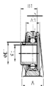
USPE200
