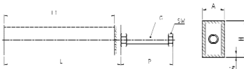
SPR1+2
