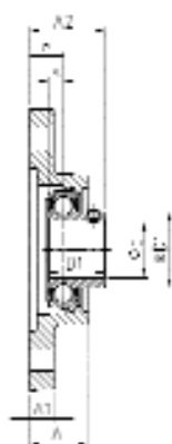
USFL200
