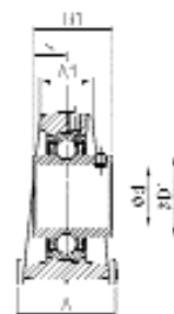
UCPAE200
