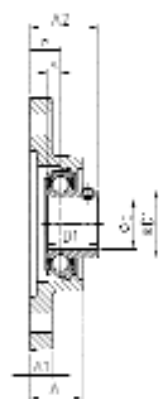
USFL200
