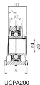
UCPA200
