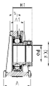
ESPA200
