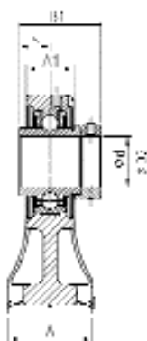
EXPH200
