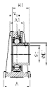
USPA200
