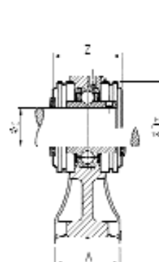
UCPH200CO(CC)
