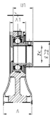
ESPH200
