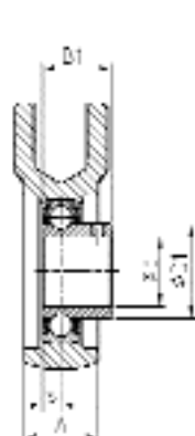
USEHE200
