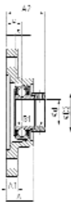
ESFL200
