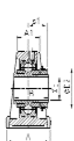
UKPAE200H
