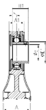
USPH200
