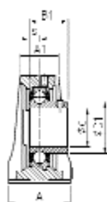
USP200
