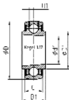
UK200
