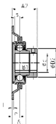
ESPFE200
