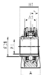
UCPE200
