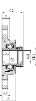
EXFL200 EXFL300
