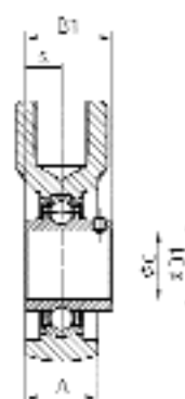
UCEHE200
