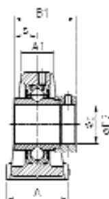
EXP200
