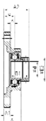
ESFLE200
